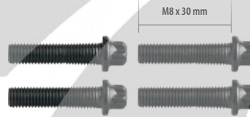
CC65097 Bolt
