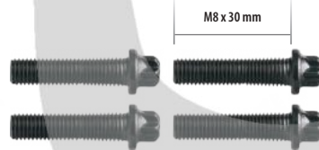
CC65097 Bolt
