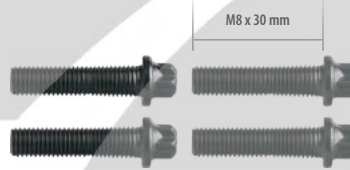
CC65097 Bolt
